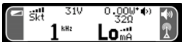
Figur 22 – LO-strøm (low output – lav utgang)
