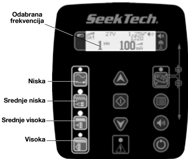
Slika 19 – Gumbi za frekvenciju – Prijemnik/lokator drugog proizvođača
