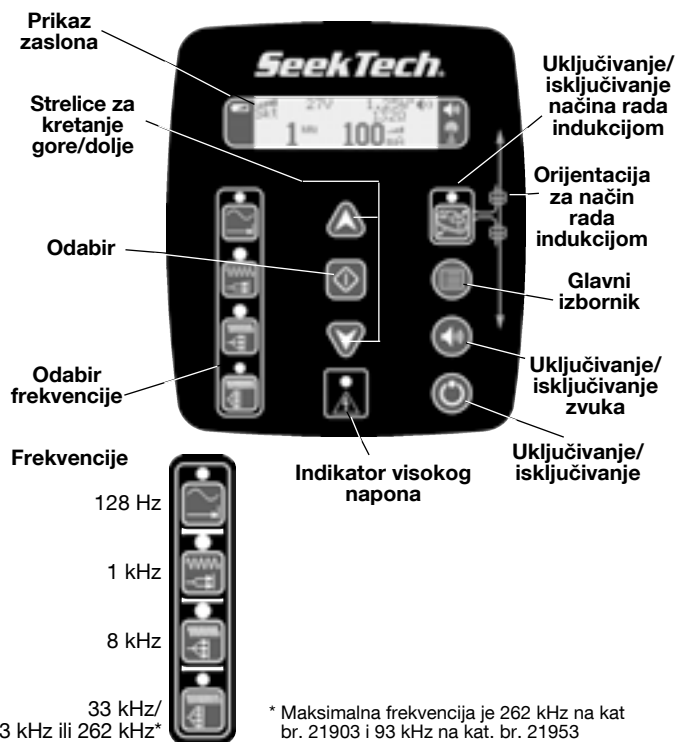
Slika 4 – Tipkovnica
