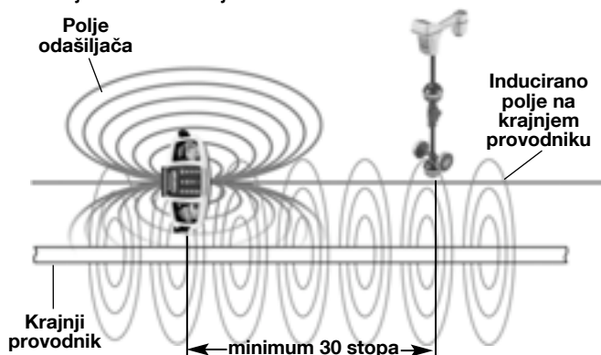
Slika 15 – U načinu rada indukcijom locirajte najmanje na 30 stopa od odašiljača, kako biste osigurali praćenje krajnjeg provodnika
