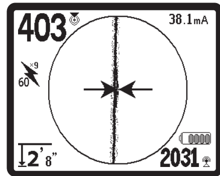
Рис. 29: Использование 9-ой гармоники частоты 60 Гц для пассивного обнаружения трассы магистрالی
