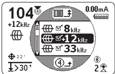
图 13 – 活动自定义频率
