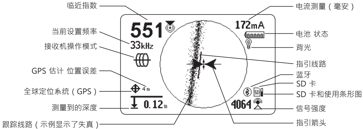
图 1 - 线路跟踪模式显示示例
