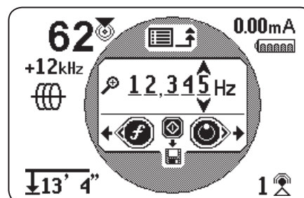
图 12 – 频率输入屏幕
