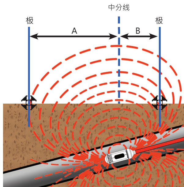
图 9 – 倾斜 RIDGID NaviTrack 电池信号发生器
