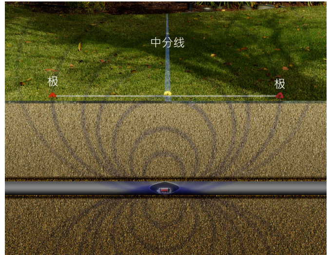
图 7 – 极和中分线位置
