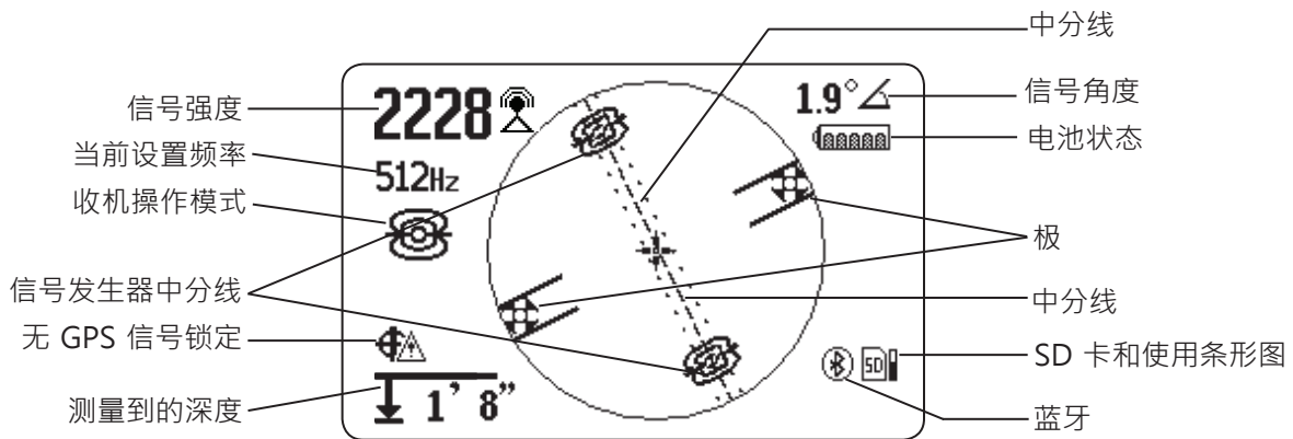
图 3 - 显示器显示了中分线和中分线信号发生器图标
