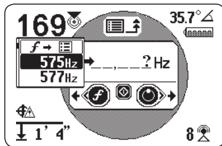
图 14 – 常用频率列表
