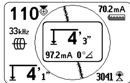
图 10 – 深度平均值报告
