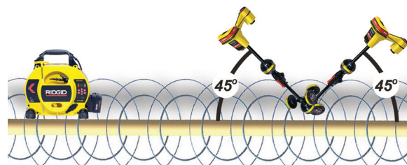
图 5 – 45° 倾斜测试
