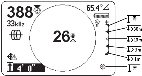
图 15 – 接近阈值控制限制设置，以显示信号强度
