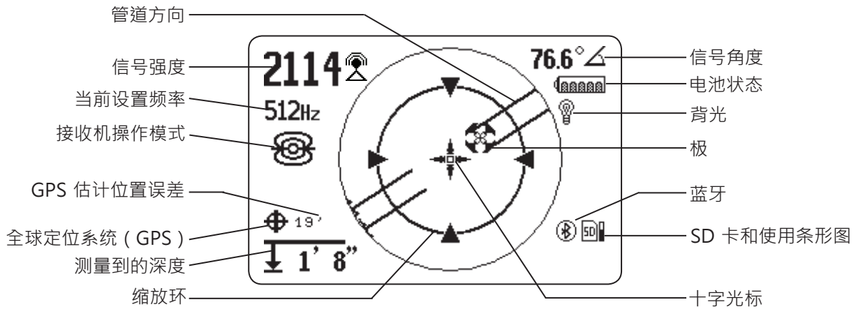
图 2 - 信号发生器模式显示示例
