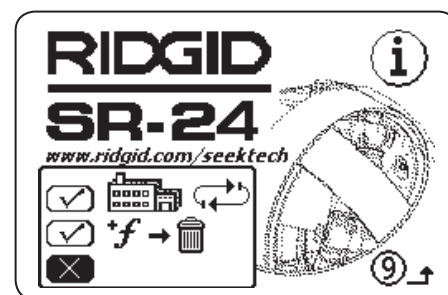
Figur 16 – Återställningsalternativ
