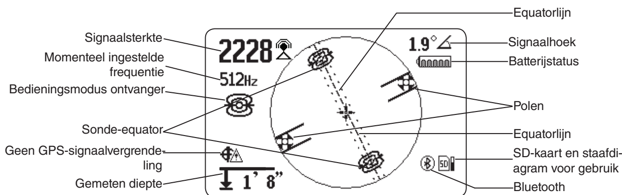
Afbeelding 3 – Weergave met pictogrammen Equatorlijn en Equatorsonde
