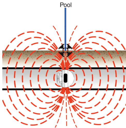
Afbeelding 8 – Drijvende RIDGID NaviTrack- FloatSonde
