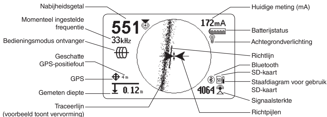
Afbeelding 1 – Voorbeeld weergave modus Leidingtracing
