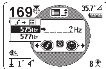
Figura 14 – Lista delle frequenze di uso frequente
