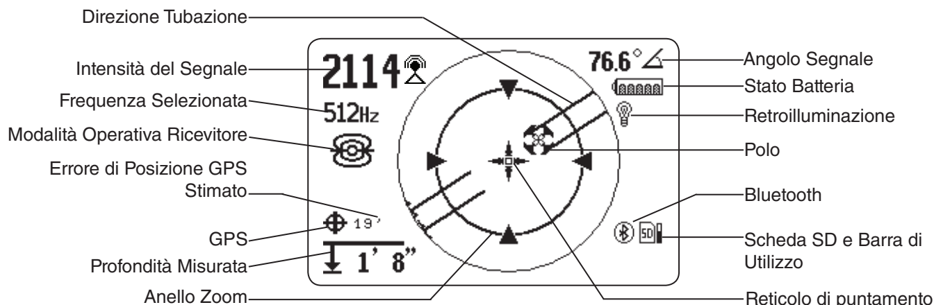
Figura 2 – Esempio Display Modalità Sonda
