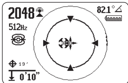
Figura 6 – Centrare i Poli nel Reticolo di Puntamento
